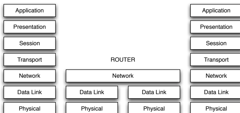
Figura 1.9: Instradamento a livello 3 mediante un router
